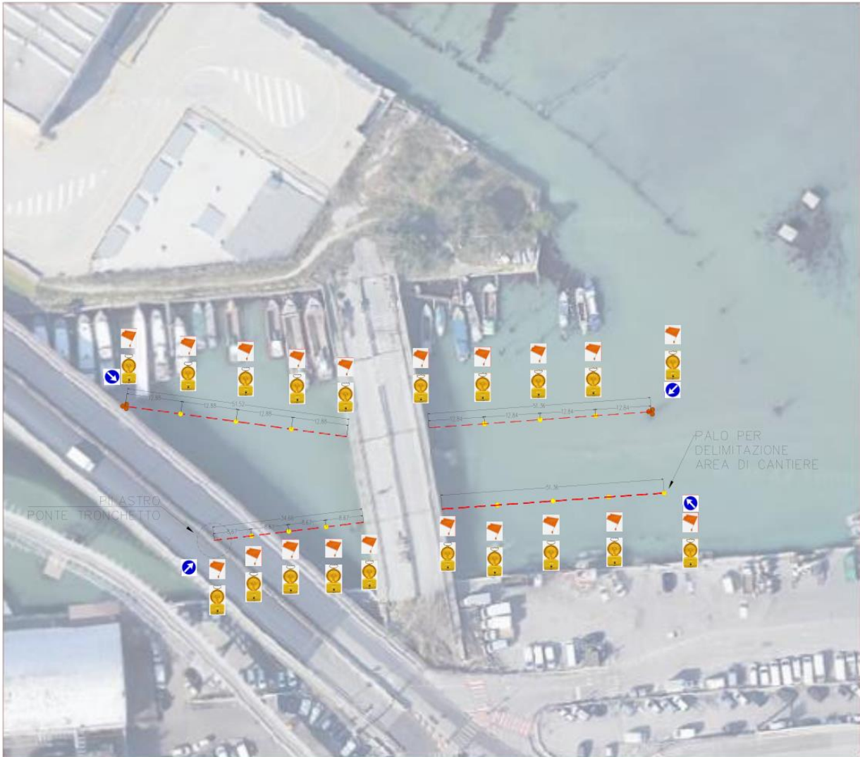
PONTE DISMESSO SU CANALE COLOMBUOLA DELIMITAZIONE AREA CANTIERE CON OPPORTUNA SEGNALETICA-VISTA PIANTA
